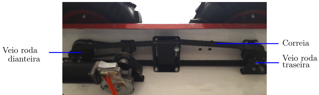
Figura 2.2: Sistema de transmissão utilizado na plataforma
