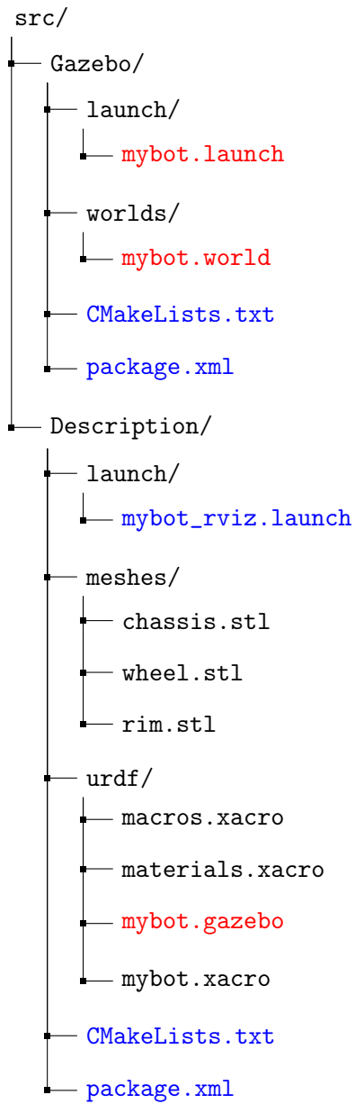
Figura 5.5: Esquema de ficheiros final para o ambiente de simulação virtual, estando a azul os ficheiros somente utilizados pelo ROS, a vermelhos os ficheiros somente usados pelo Gazebo, e os que são usados por ambos a preto
